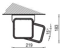
Installazione a soffitto 15° 15° ceiling installation
