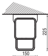
Installazione a soffitto 90° 90° ceiling installation
