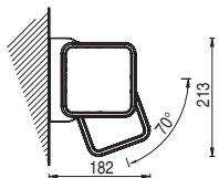
Installazione a parete 70° 70° wall installation
