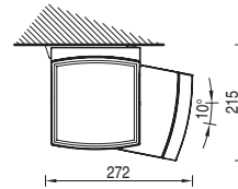
Installazione a soffitto 10° 10° ceiling installation
