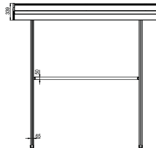
Vista dall'alto (2 profili guida) Top view (2 guide profiles)
