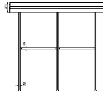
Vista dall'alto (3 profili guida) Top view (3 guide profiles)
