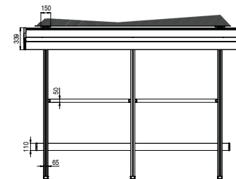
Vista dall'alto (3 profili guida) Top view (3 guide profiles)
