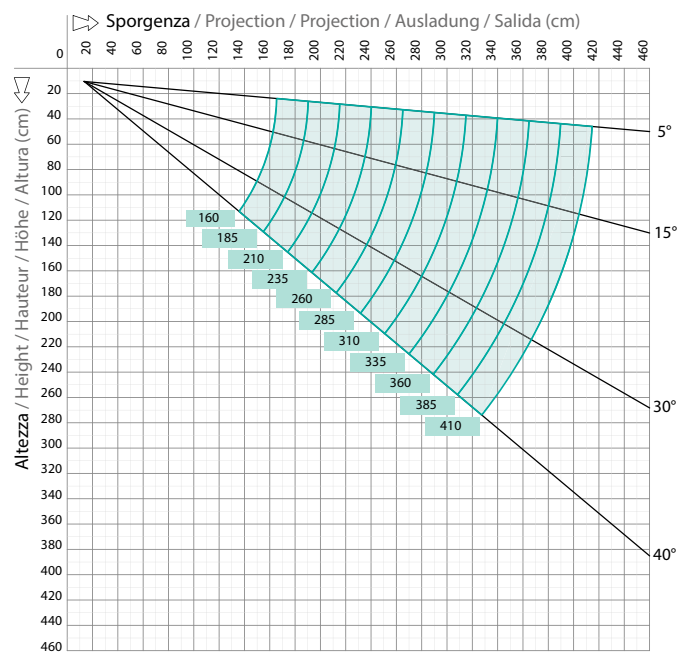
Diagramme de couverture - Installation façade
