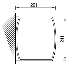
Installazione a parete con terminale a cassonetto. Wall installation with box front bar
