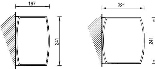
Installazione a parete Wall installation
