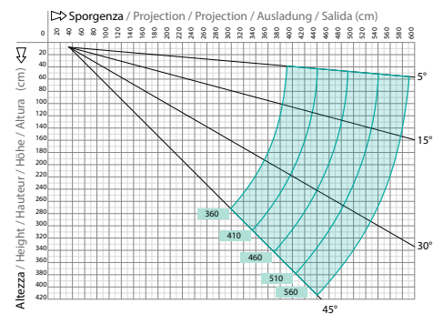
Diagramma di copertura - Installazione a soffitto Covering diagram - Ceiling installation
