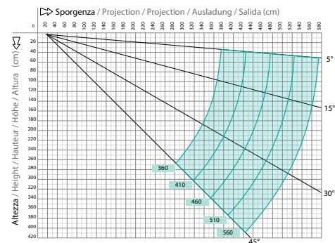
Diagramma di copertura - Installazione a parete Covering diagram - Wall installation
