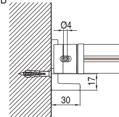
floor bracket - pie suelo B-B
