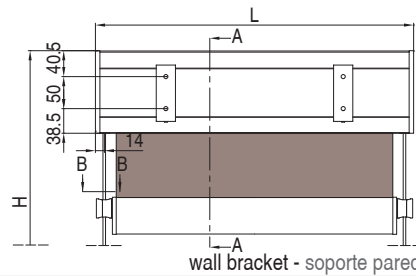
rear view - vista posterior
