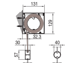
SQUARE - CUADRO A-A
