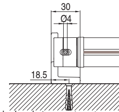
niche bracket - soporte entraparedes B-B
