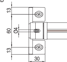
floor bracket - pie suelo B-B
