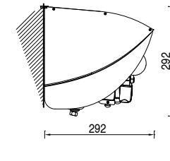
Installation with hood Montaje con tejadillo
