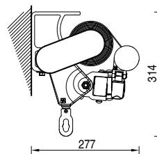
Installazione a parete con staffa estrusa. Wall installation with extruded bracket
