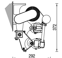
Installazione con bracci incrociati. Cross arms installation
