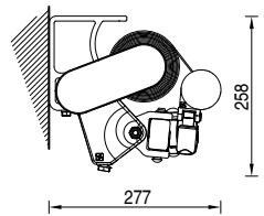
Installazione a soffitto con staffa estrusa. Ceiling installation with extruded bracket
