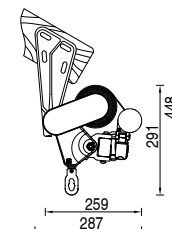
Installazione con bracci incrociati. Cross arms installation
