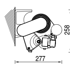
Installazione a parete Wall installation
