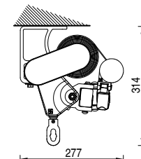
Installazione a soffitto con staffa estrusa. Ceiling installation with extruded bracket
