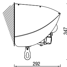
Installazione con tettuccio Installation with hood
