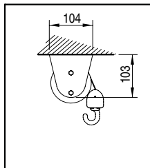
Installazione a soffitto con culla Ceiling installation with concave support
