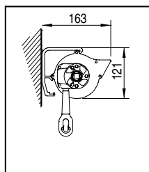
Installazione a parete Wall installation
