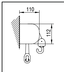
Installazione a parete Wall installation
