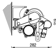
Installazione a parete versione Gold Wall installation Gold version
