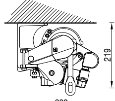
Installazione a soffitto versione Gold Ceiling installation Gold version
