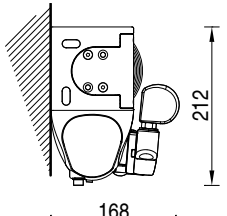
Installazione a parete Wall installation
