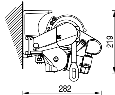
Installazione a parete versione Gold Wall installation Gold version
