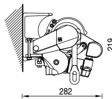
Installazione a parete versione Gold Wall installation Gold version
