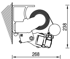
Installazione a parete con staffa estrusa. Wall installation with extruded bracket
