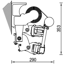
Installazione con bracci incrociati. Cross arms installation
