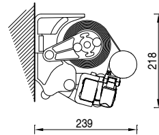
Installazione a parete Wall installation
