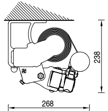
Installazione a soffitto con staffa estrusa. Ceiling installation with extruded bracket
