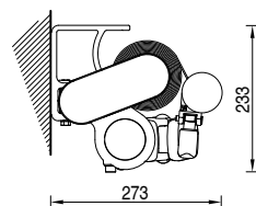
Installazione a parete con staffa estrusa. Wall installation with extruded bracket
