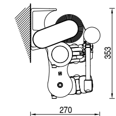
Installazione con bracci incrociati. Cross arms installation
