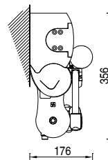
Installazione a parete con bracci incrociati Crossed arms installation
