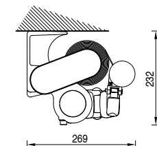
Installazione a soffitto con staffa estrusa. Ceiling installation with extruded bracket
