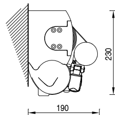
Installazione a parete Wall installation
