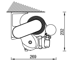
Installazione a soffitto con staffa estrusa. Ceiling installation with extruded bracket
