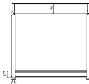
Vista dall'alto (modulo singolo) Top View (single module)
