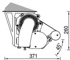
Installazione a soffitto 45° 45° ceiling installation
