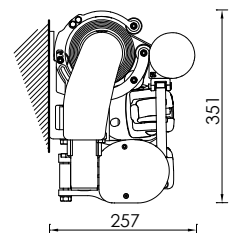
Installazione con bracci incrociati Crossed arms installation
