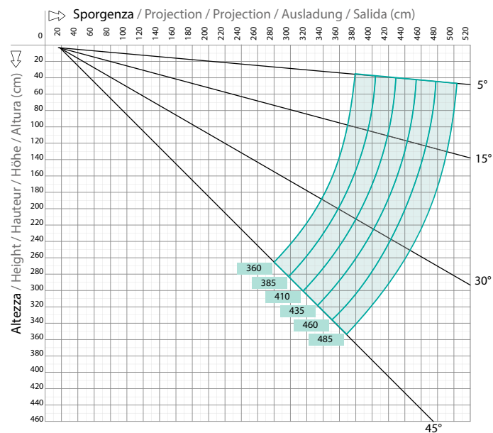
Diagramma di copertura - Installazione parete/soffitto Covering diagram - Wall/ceiling installation
