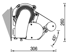
Installazione a parete 45° 45° wall installation
