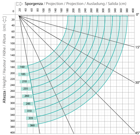
Diagramme de couverture - installation façade
