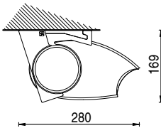
Installation plafond
