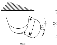
Installation plafond 15°
