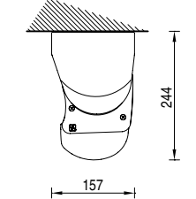
Installation plafond 90°
