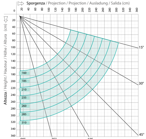
Diagramme de couverture - installation plafond
