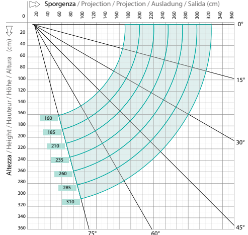
Diagramme de couverture - installation façade
