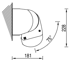
Installazione a parete 75° 75° wall installation
