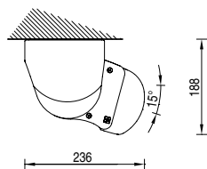
Installazione a soffitto 15° 15° Ceiling installation
