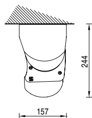
Installazione a soffitto 90° 90° ceiling installation
