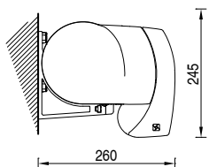
Installazione a parete con terminale a cassonetto Wall installation with box front bar
