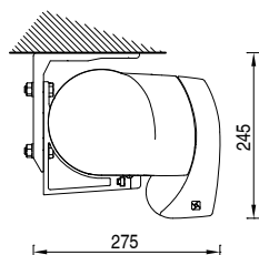
Installazione a soffitto con terminale a cassonetto Ceiling installation with box front bar
