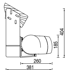
Installazione sottotetto Under-roof installation
