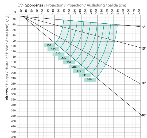
Diagramma di copertura - Installazione a parete/soffitto Covering diagram - Wall/ceiling installation
