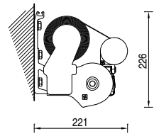
Installazione a parete Wall installation
