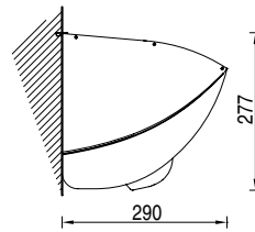
Installazione con tettuccio. Installation with hood
