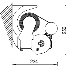
Installazione a parete con staffa parete/soffitto. Wall installation with wall/ceiling bracket
