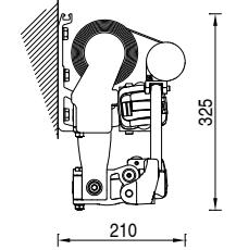
Installazione con bracci incrociati. Crossed arms installation
