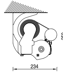
Installazione a soffitto con staffa parete/soffitto. Ceiling installation with wall/ceiling bracket
