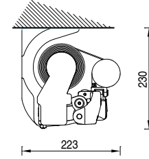
Installazione a soffitto con staffa parete/soffitto. Ceiling installation with wall/ceiling bracket
