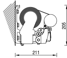
Installazione a parete Wall installation
