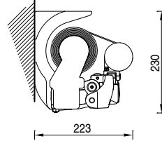
Installazione a parete con staffa parete/soffitto. Wall installation with wall/ceiling bracket
