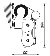
Installazione con bracci incrociati. Crossed arms installation
