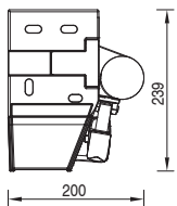
Installazione a nicchia Niche installation
