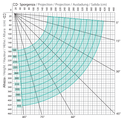
Diagramma di copertura - Installazione a parete/soffitto/ nicchia Covering diagram - Wall installation/ceiling/niche
