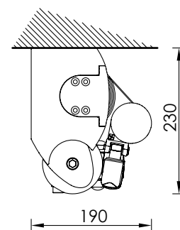
Montaggio a soffitto Ceiling installation
