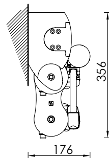
Montaggio con kit bracci incrociati Installation with crossed arm kit
