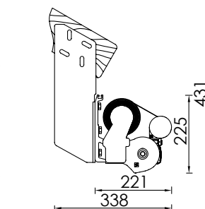
Montaggio sottotetto Under-roof installation
