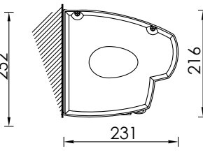
Montaggio sottotetto Under-roof installation
