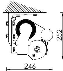
Montaggio a soffitto con staffa universale Ceiling installation with universal bracket
