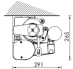
Montaggio a soffitto Ceiling installation
