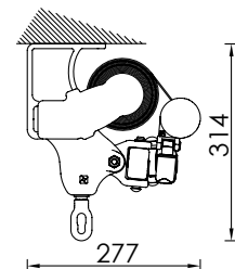
Montaggio a soffitto con staffa estrusa Ceiling installation with extruded bracket
