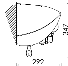
Montaggio con tettuccio Installation with a hood
