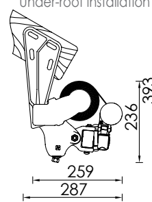
Montaggio sottotetto Under-roof installation
