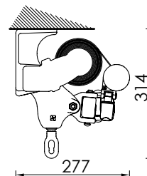
Montaggio a soffitto Ceiling installation
